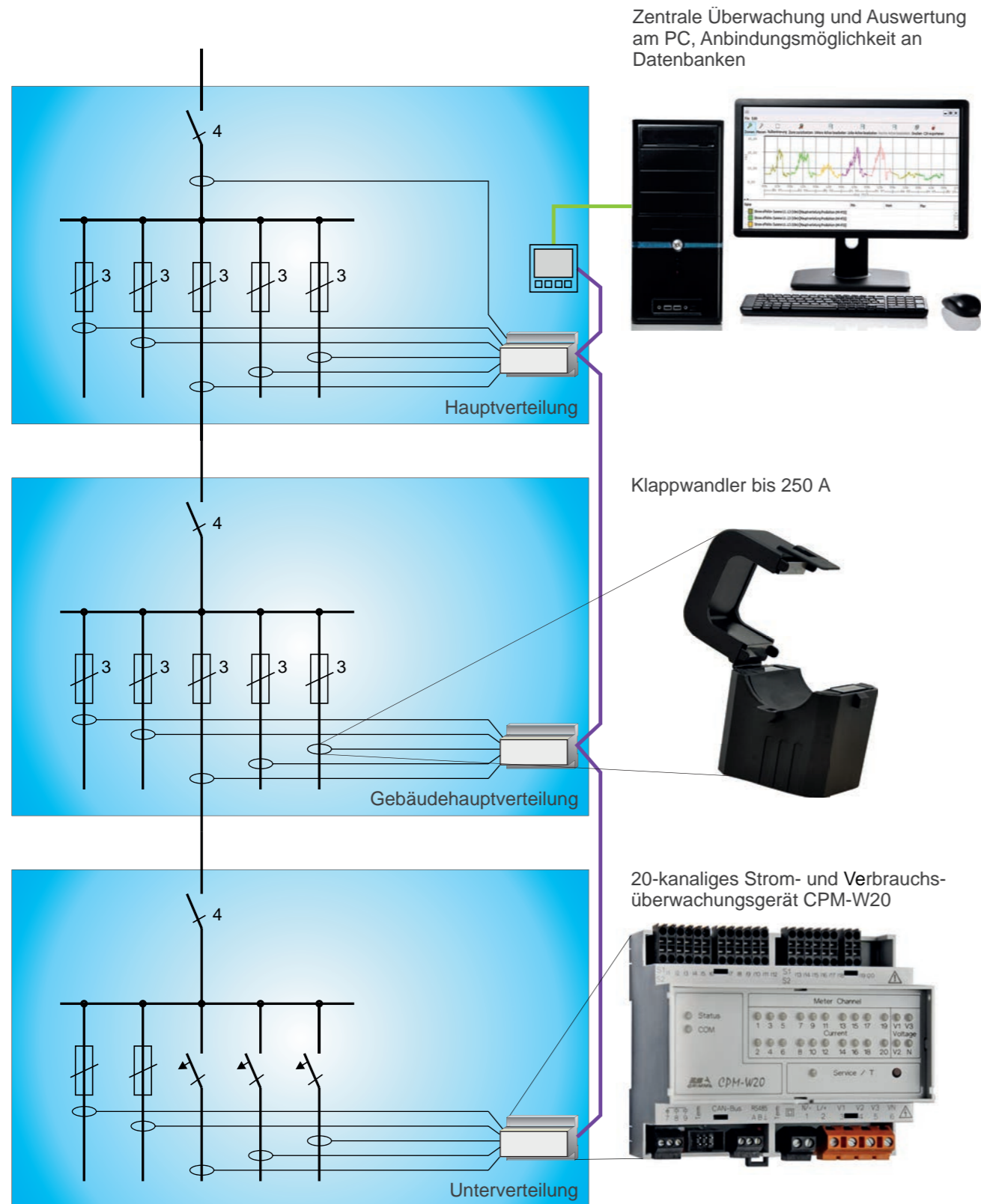
Prinzipdarstellung einer Energieverbrauchserfassung in einem Krankenhaus (dargestellt ist die AV-Seite)
