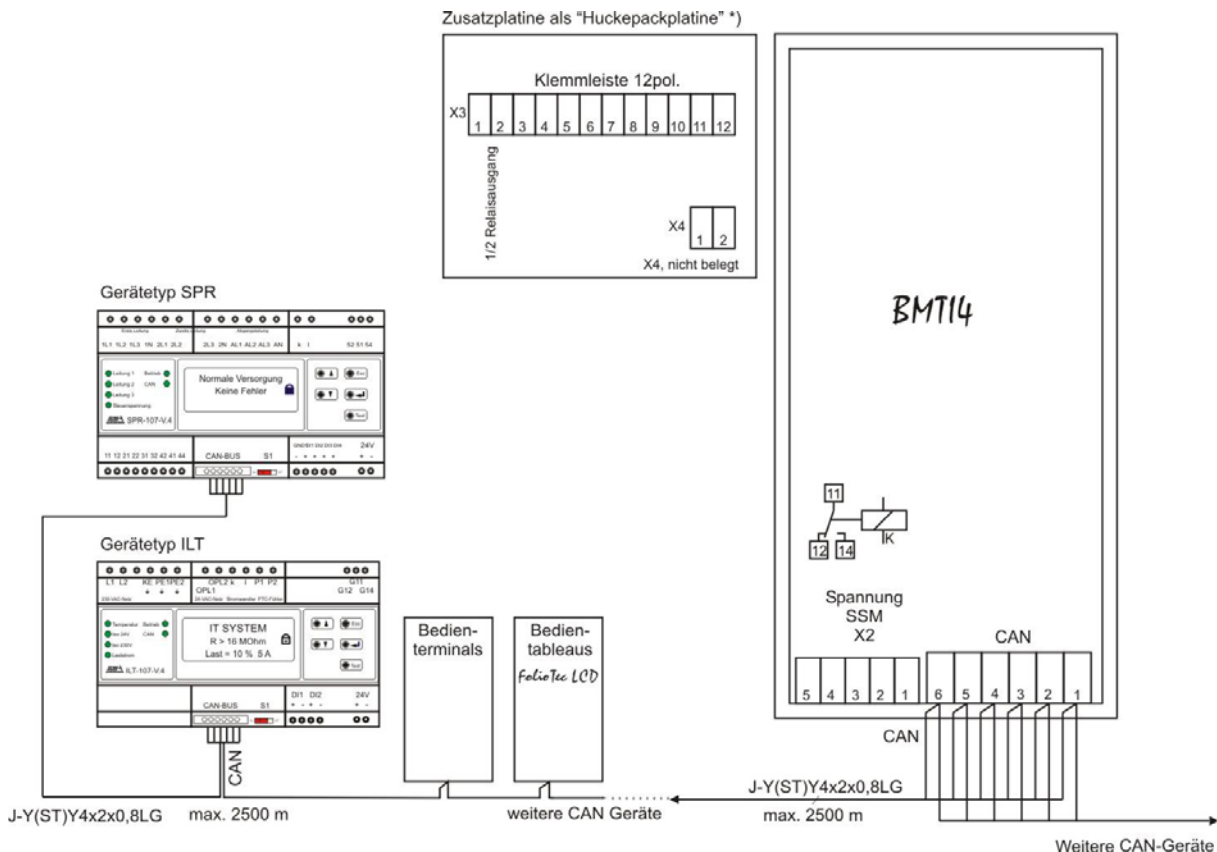
Abb. 1: Anschlussschaltbild
