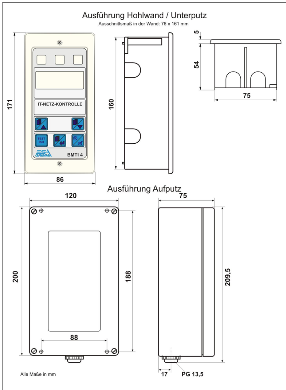
Abb. 2: Geräteabmessungen
