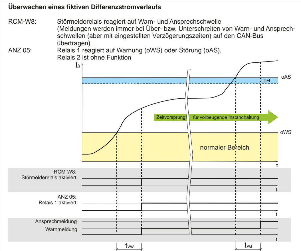
Abb. 4: Fiktiver Differenzstromverlauf
