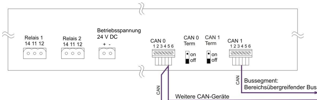
Abb. 6: Anschlussschaltbild
