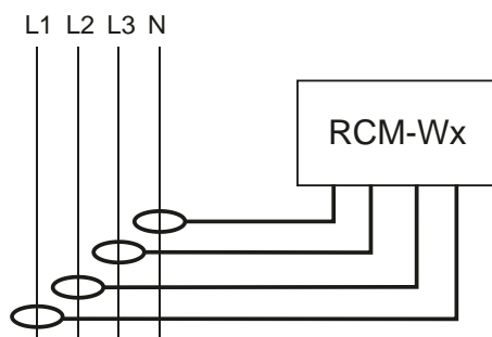
Abb. 1: Vereinfachte Darstellung einer Betriebsstrommessung
