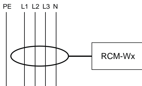
Abb. 2: Vereinfachte Darstellung einer Differenzstrommessung
